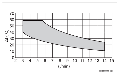
Obr. 31 14litrový model
