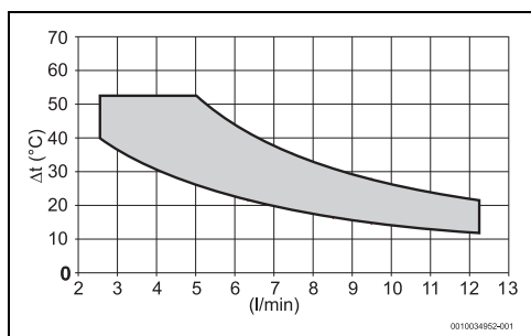
Obr. 30 11 litrový model
