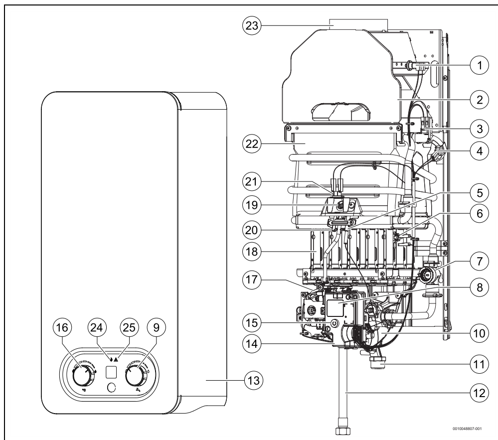
Obr. 2 Konstrukce zařízení
