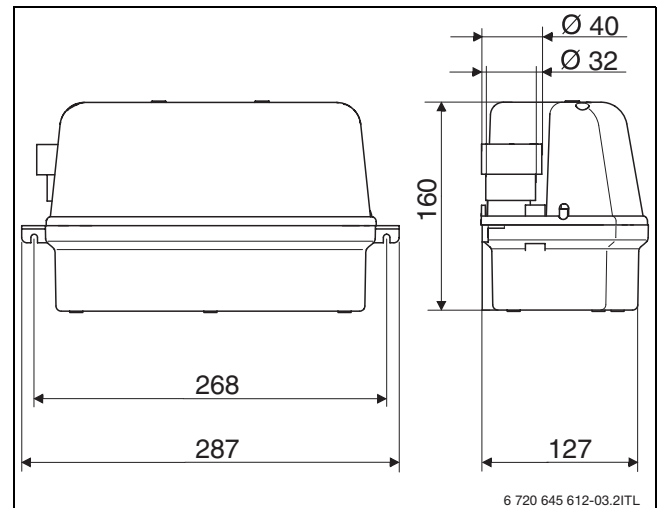
Afb. 2 Afmetingen
