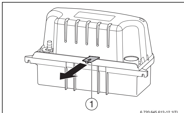
Fig. 6 Înlăturarea siguranței
