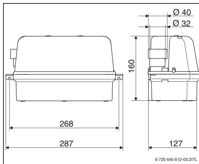
Bild 2 Abmessungen
