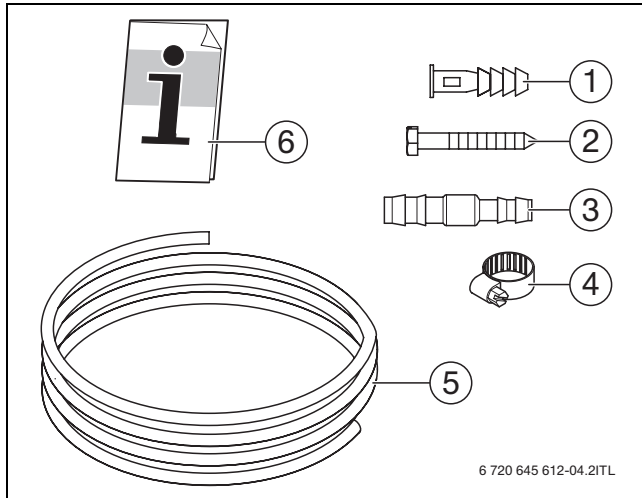
Şekil 1 Teslimat kapsamı
