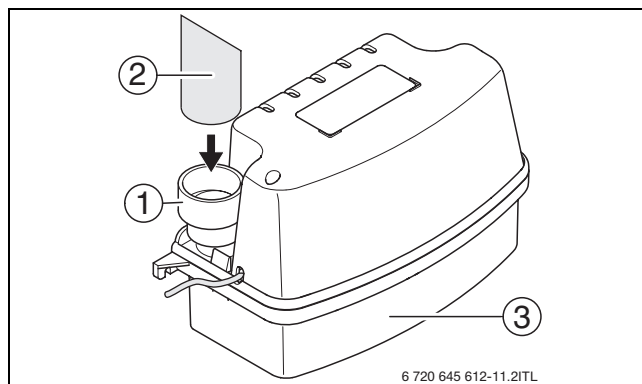
Bild 7 Zulaufschlauch montieren
