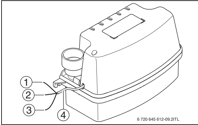
Şekil 11 Arıza gösterge sisteminin telleri
