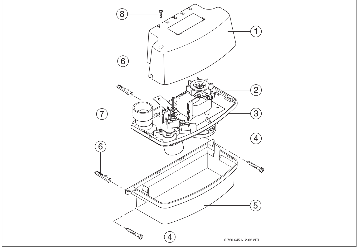
Şekil 4 Yoğuşma suyu pompasının yapısı
