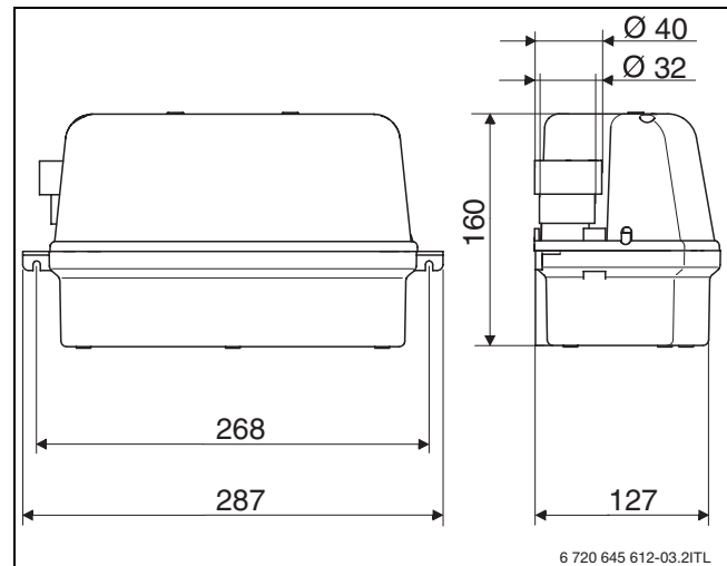
Fig. 2 Dimensioni
