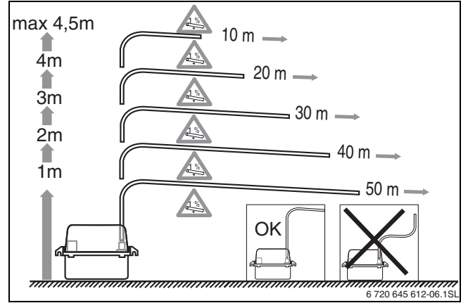
Şekil 10 Tahliye hortumunun monte edilmesi
