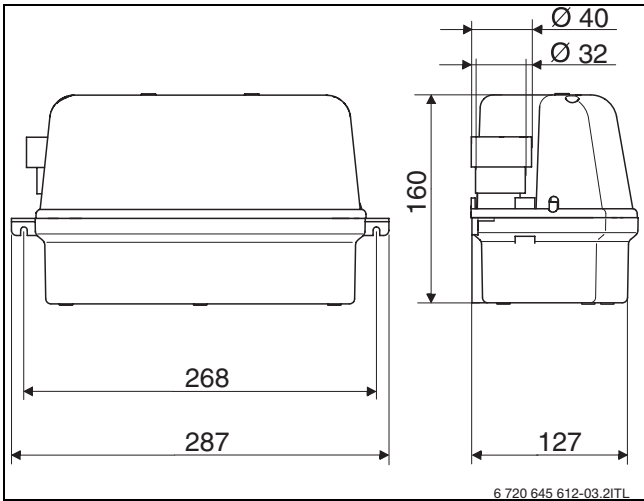
Fig. 2 Dimensions
