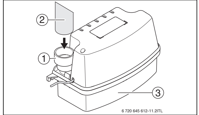
Şekil 7 Giriş hortumunun monte edilmesi
