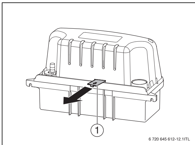
Bild 6 Sicherung entfernen
