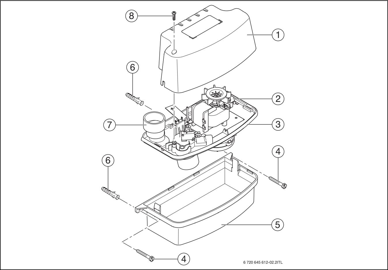
Afb. 4 Constructie condensafvoerpomp
