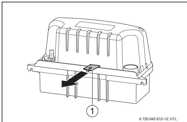
Fig. 6 Retirar protección
