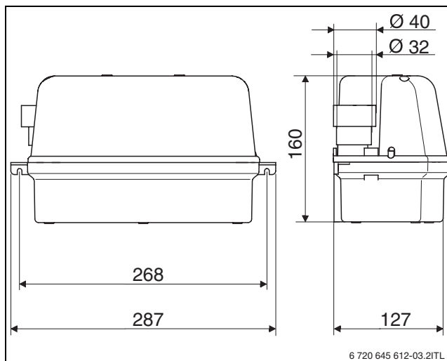
Fig. 2 Dimensiuni
