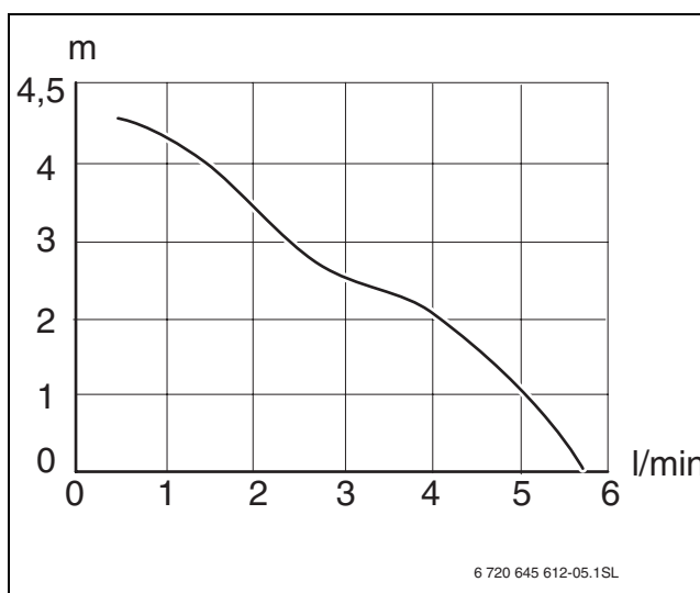
Rys. 3 Wydajność pompy (l/min) w zależności od wysokości podnoszenia
