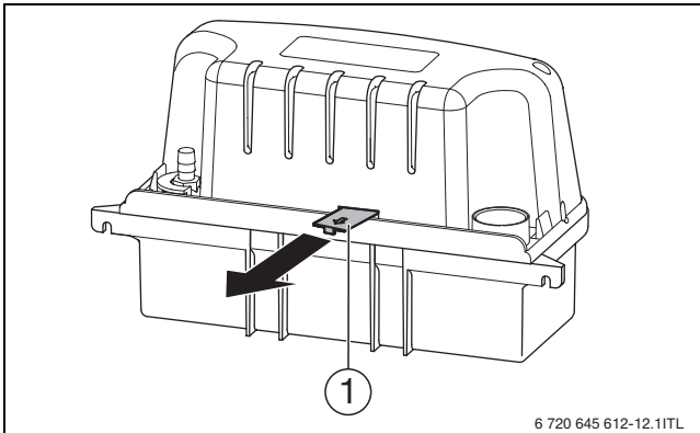
Şekil 6 Sigortanın sökülmesi
