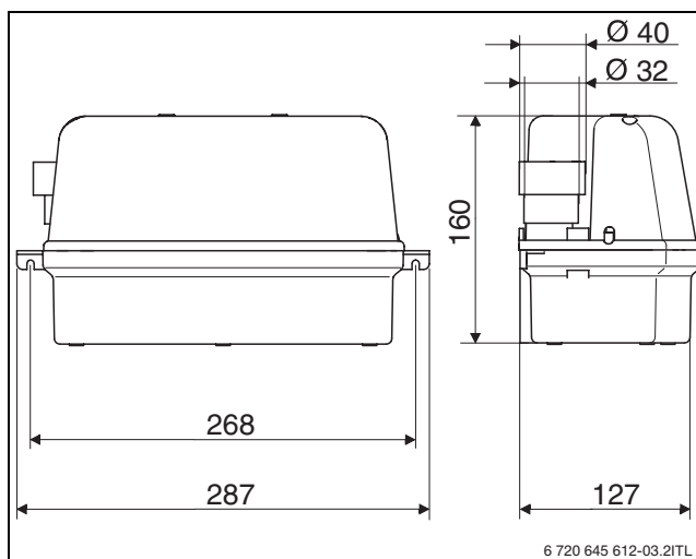
Rys. 2 Wymiary
