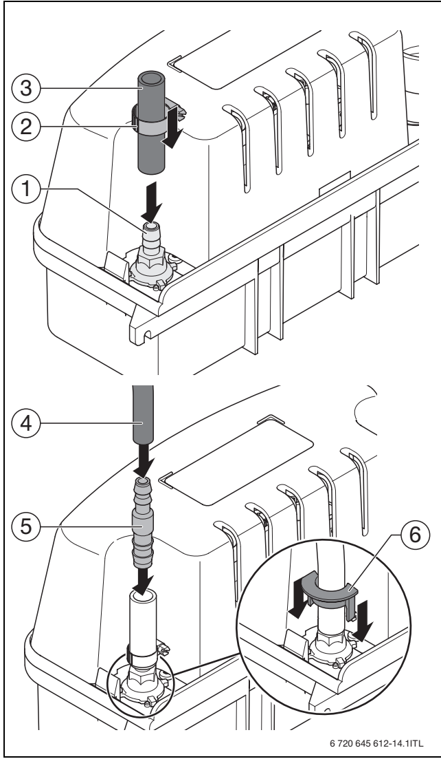
Şekil 9 Tahliye hortumunun adaptörle monte edilmesi
