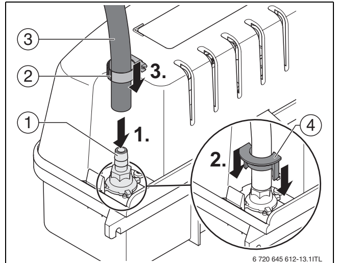
Şekil 8 Tahliye hortumunun monte edilmesi
