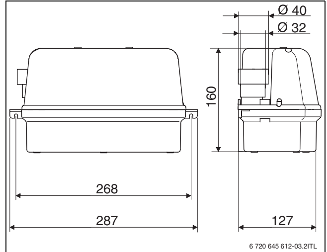
Şekil 2 Boyutlar
