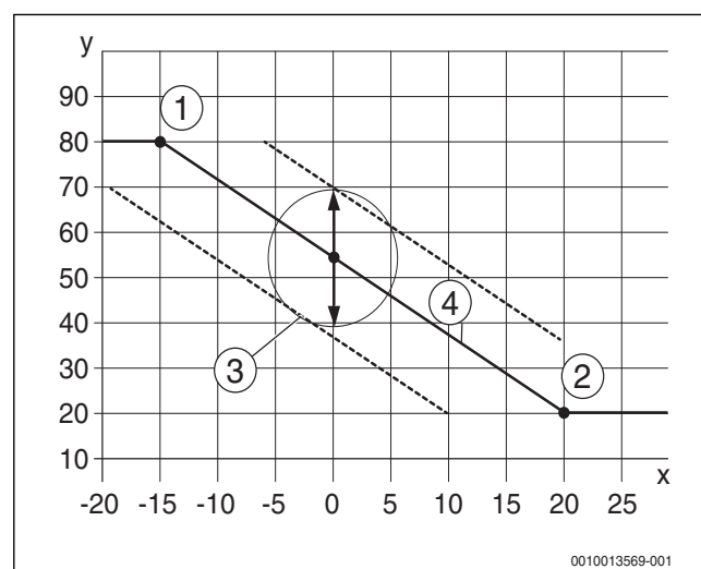
Obr. 4 Ekvitermní křivka
