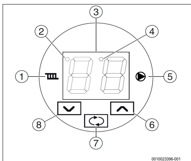
Obr. 3 Ovládací panel modulu KASK - 230
