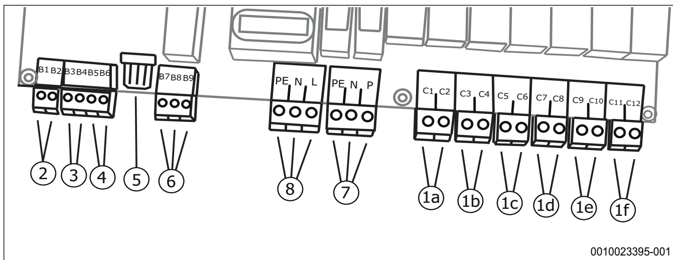
Obr. 2 Zapojení konektorů modulu KASK - 230
