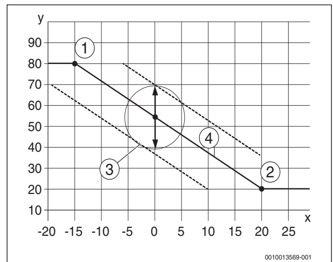
Obr. 4 Ekvitermní křivka
