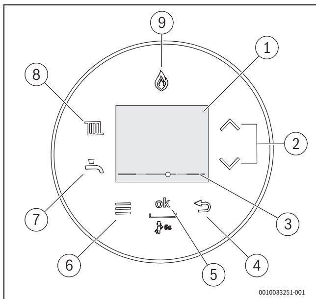
Obr. 2 Ovládací panel
